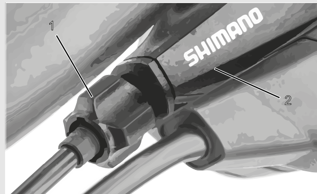
Afbeelding 37: Afstelwartel (1) van de versnelling met enkele bowdenkabelbediening en behuizing van de schakelhendel (2), voorbeeld
