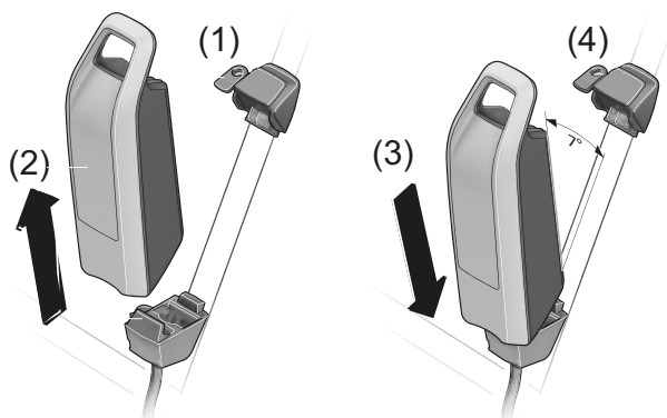
Afbeelding 28: Frame-accu verwijderen en aanbrengen
