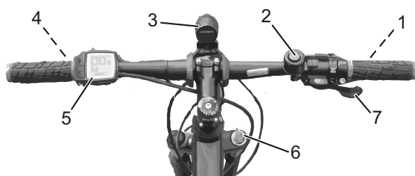
Afbeelding 11: Detailaanzicht pedelec vanuit berijderpositie gezien, voorbeeld
