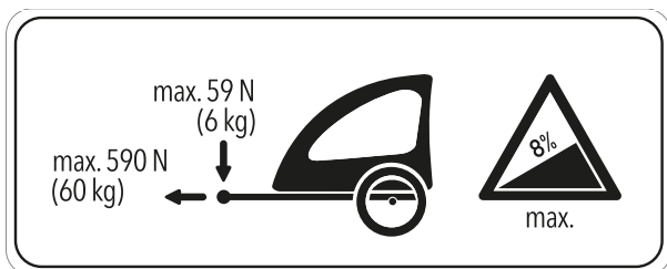
Afbeelding 27: Waarschuwingsticker aanhanger
