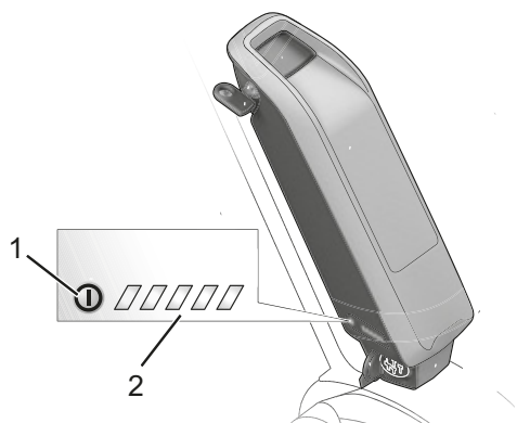
Afbeelding 12: Voorbeeld laadtoestandweergave
