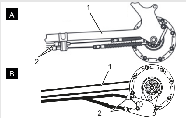
Afbeelding 38: Afstelwartels (2) van twee alternatieve uitvoeringen (A resp. B) van een versnelling met dubbele bowdenkabelbediening aan de achterbrug (1)
