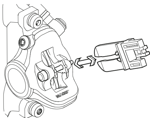
Afbeelding 14: Transportbeveiliging bevestigen
