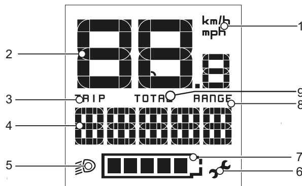
Afbeelding 13: Overzicht displayweergaven
