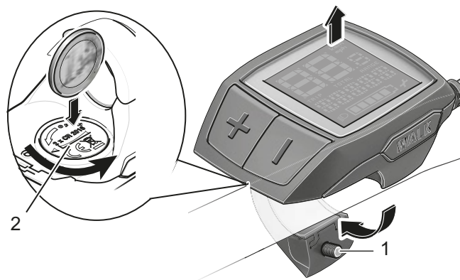
Afbeelding 30: Display met bevestigingsschroef (1) en deksel (2) van het batterijcompartiment
